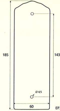
demi plaque Anglaise
