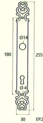
Manoir larg. réd.
